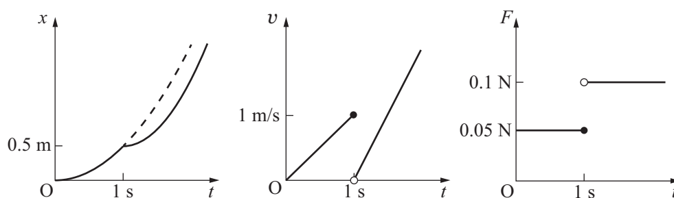
図 2: 問題 2.2-1 の質点の位置座標, 速度, 働く力
