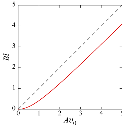
図 7: 式 (16) で表される, バネの最大縮み l と物体がバネに接触する瞬間の速さ v_0 との関係 (実線). ただし, A = \sqrt{k/m/g\mu'} , B = k/mg\mu' とおいた. 破線は摩擦がない場合 ( \mu' = 0 ) の結果を表す,
