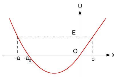
図 4: ポテンシャル U(x) のグラフ。 x > 0 の領域では直線、 x < 0 では放物線である。
