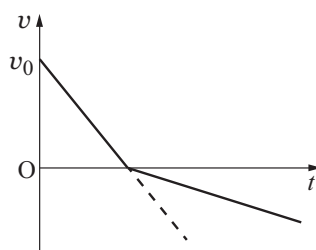
図 6: 問題 4.2-1 の状況 (2) における，物体の速度 v と時間 t の関係．
