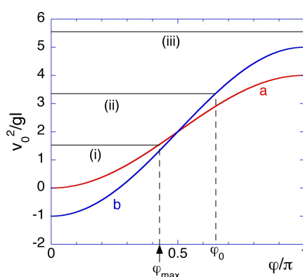
図 5: 曲線 a と b はそれぞれ、不等式 (13) と (14) の右辺の関数のグラフである．
