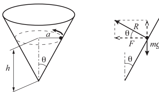
図 3: 問題 2.2-2 の運動のようすと, 質点に働く力
